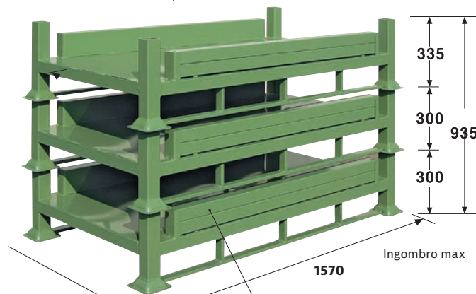
ALLOGGIO DEI MONTANTI ASPORTABILI
