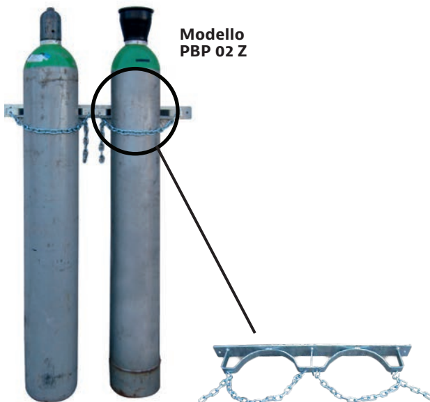
Supporto a parete nr. 2 bombole
